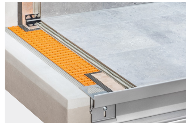
Konstrukcja balkonu z uszczelnieniem zespolonym Schlüter-DITRA
