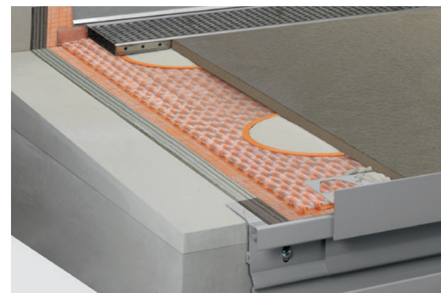
Układanie płyt na Schlüter-KERDI i Schlüter-TROBA-PLUS 8G z zastosowaniem pierścieni Schlüter-TROBA-STELZ
