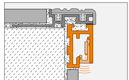
Diffusiescherm Schlüter-LIPROTEC-VBI
