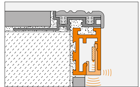
Diffusiescherm Schlüter-LIPROTEC-PBD
