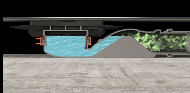
Sifone antiodore permanente grazie alla forma sinusoidale
