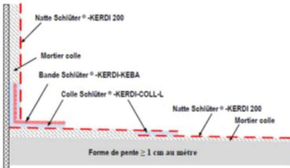
Figure 7 - Traitement d'un angle de douche avec SCHLÜTER KERDI 200 et SCHLÜTER KERDI KEBA
