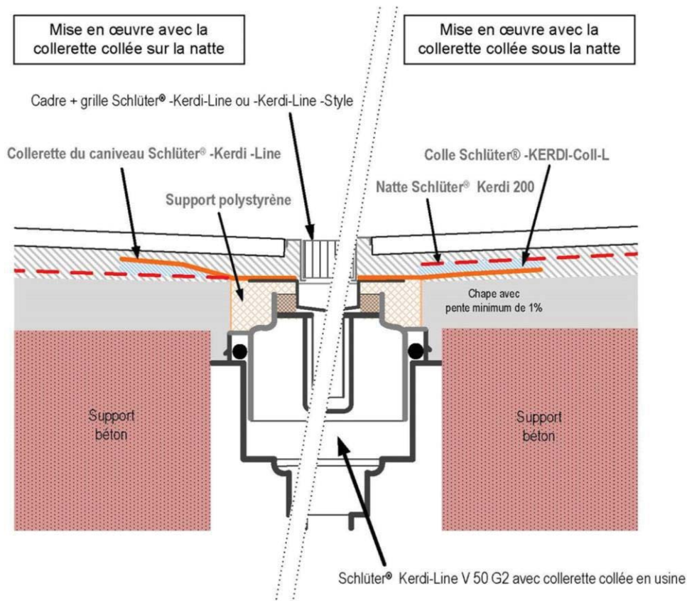
Figure 9 - Mise en œuvre du caniveau SCHLÜTER KERDI LINE V 50 G2 au centre de la douche
