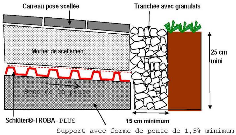
Cas b - Traitement d'un chant sur terre-plein
