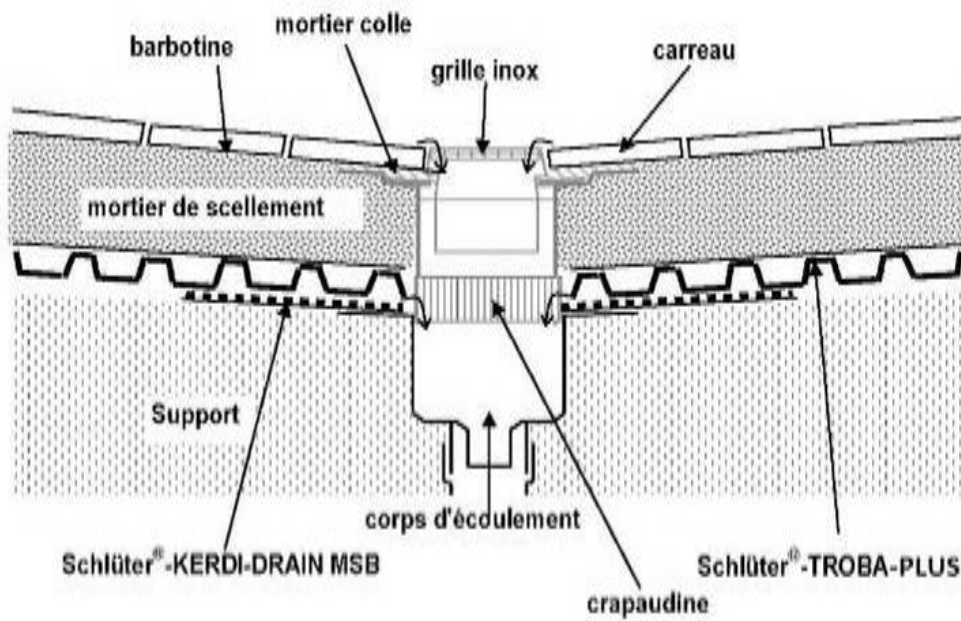
Figure 6 - Traitement des systèmes d'évacuation par siphon
