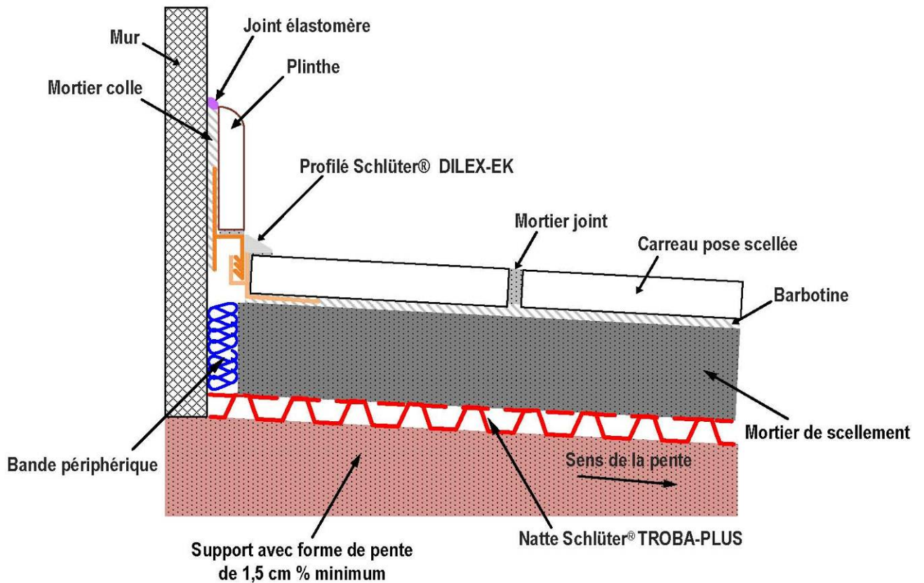
Cas c – Traitement sol-mur avec profilé d'angle SCHLÜTER DILEX EK
