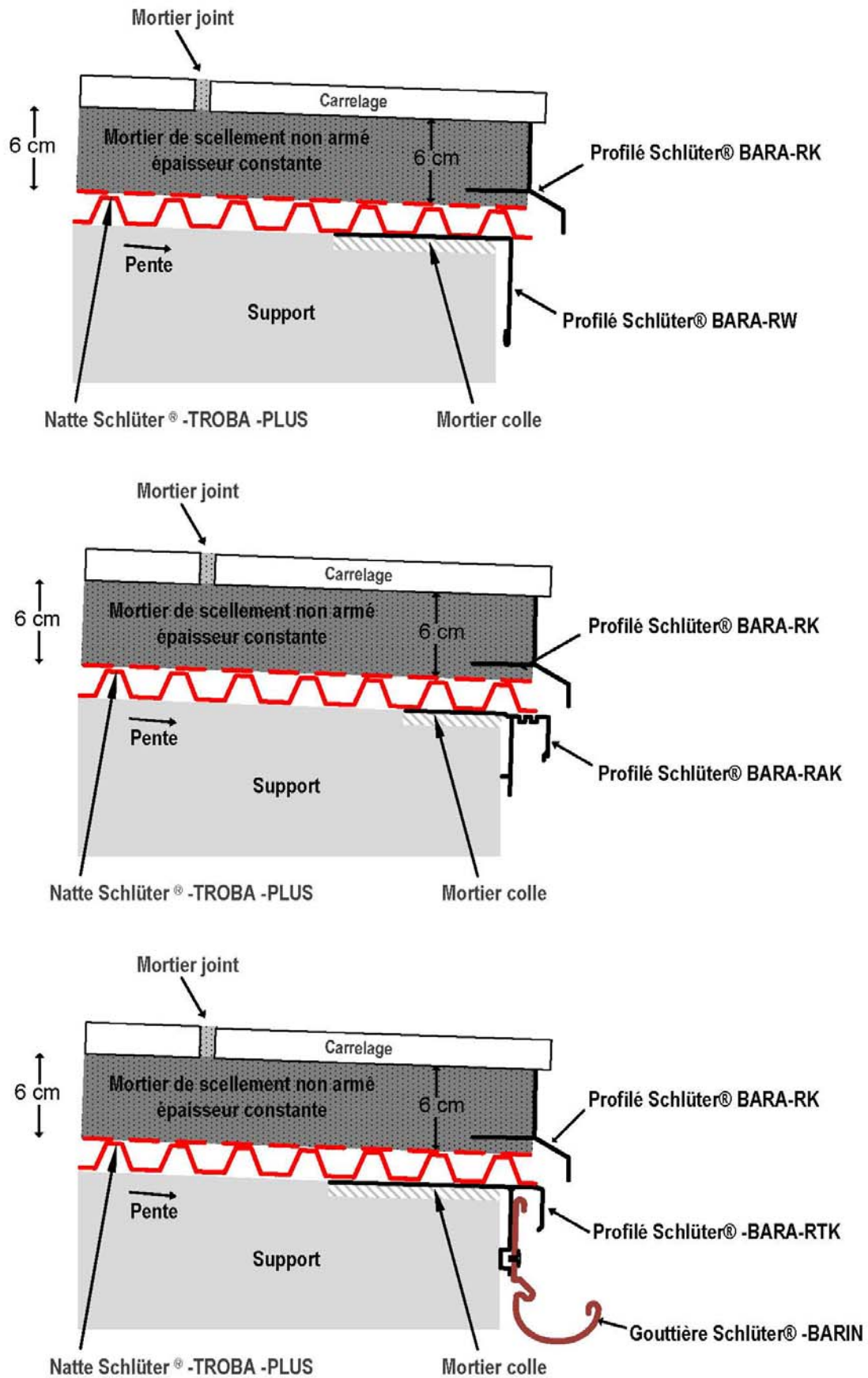
Figure 4 - Traitement des nez de balcon avec profilé de rives SCHLÜTER-BARA
