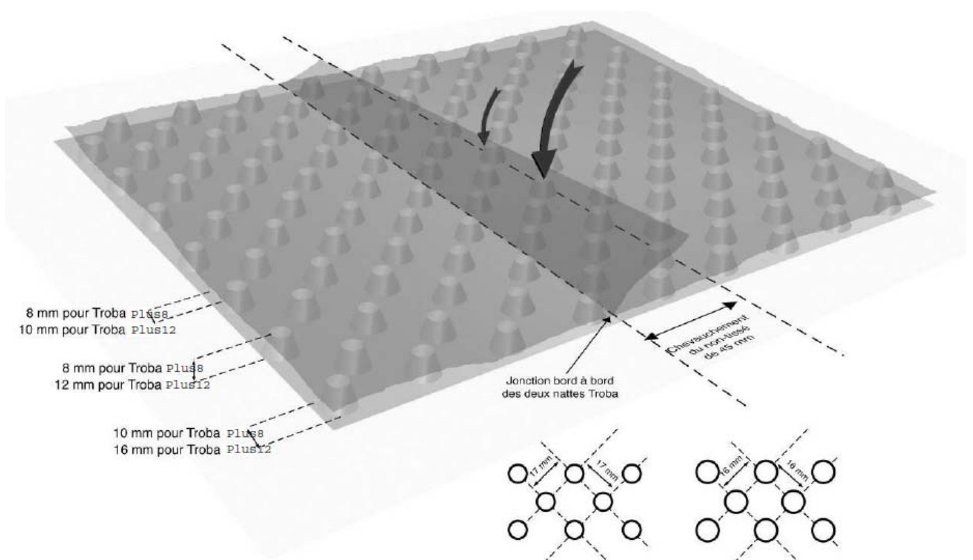
Figure 2 - Mise en œuvre de SCHLÜTER-TROBA PLUS 8 et SCHLÜTER-TROBA PLUS 12 : pose des lés bord à bord, recouvrement du non-tissé
