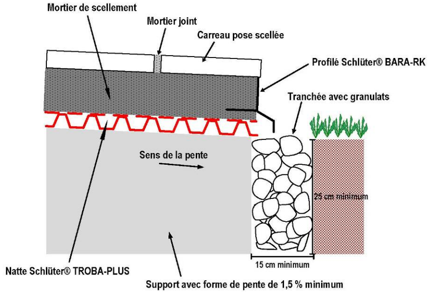
Cas b bis – Traitement d'un chant avec rives sur terre-plein
