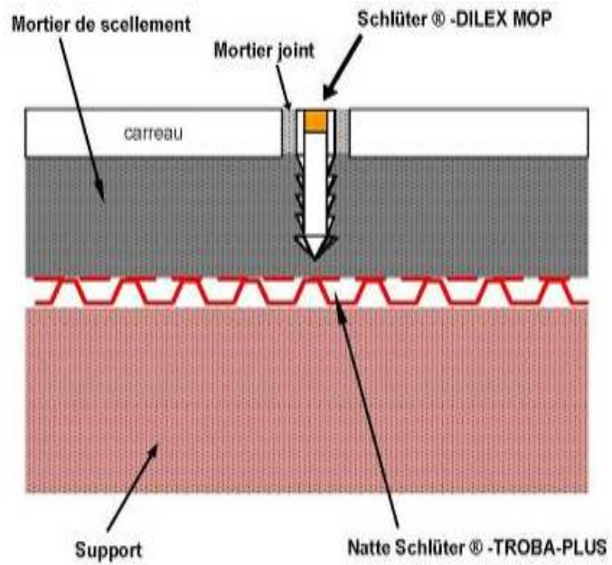
Figure 5- traitement d'un joint de fractionnement du mortier de scellement et du carrelage avec un profilé. Exemple de SCHLÜTER-DILEX-MOP
