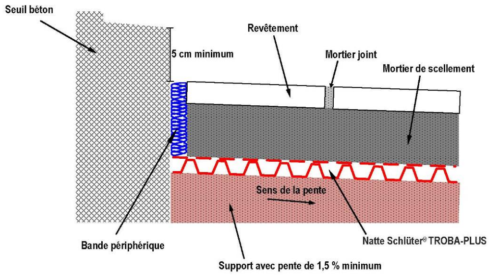
Cas a – Traitement d'un seuil
