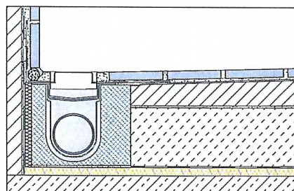
Schlüter®-KERDI-LINE-SR (Einbaubeispiel KERDI-LINE-H 40, Aufbau B siehe „Planungsgrundlagen Schlüter®-KERDI-LINE-SR“)
