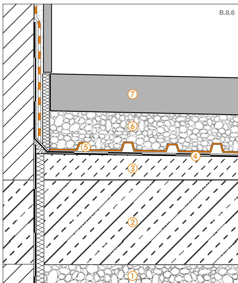
Liaison sol/mur
