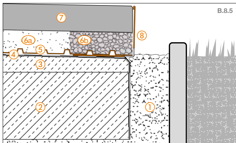
Liaison sol/mur
