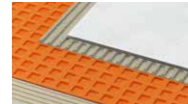
Schlüter®-DITRA 25 Lámina de desolidarización e Impermeabilización para la instalación de cerámica y piedra natural sobre soportes críticos (p. ej., yeso y soportes fisurados)
