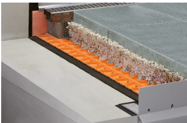
Construcción de pavimentos sobre lecho de grava/gravilla con Schlüter-TROBA
