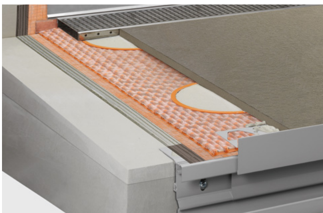
Colocación sobre Schlüter-KERDI y Schlüter-TROBA-PLUS 8G
