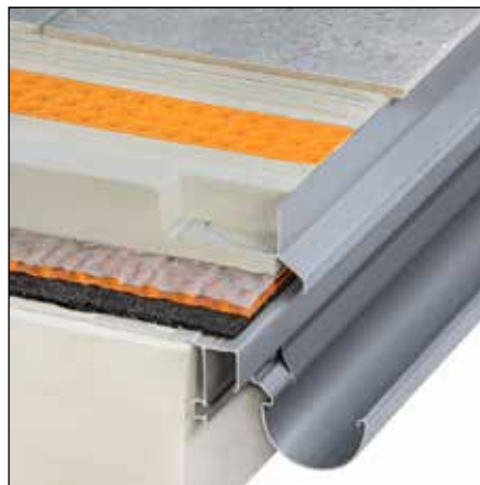
Nachträgliche Montage des Rinnensystems Schlüter®-BARIN an Randprofilen ohne Aufnahmeut
