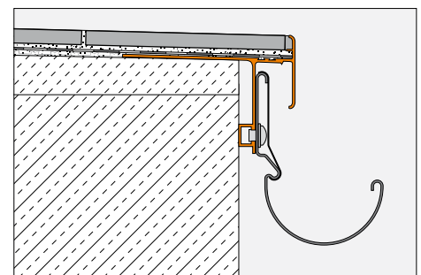
Aufbau mit Schlüter-DITRA und Schlüter-BARA-RTKEG
