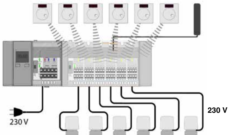
Abbildung 2: Basismodul Control, Anschlussmodul WL, Timereinheit, Raumsensor WL, externer Antenne und Stellantriebe
