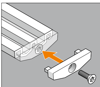
2a. Die zugehörigen Endkappen sind zu montieren
