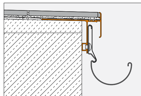
Skladba se Schlüter®-DITRA a Schlüter®-BARA-RTKEG
