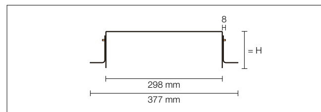
298 x 1198 mm
