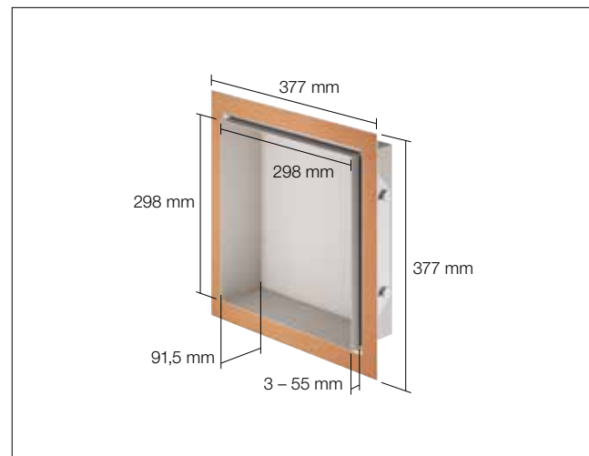
298 x 298 mm
