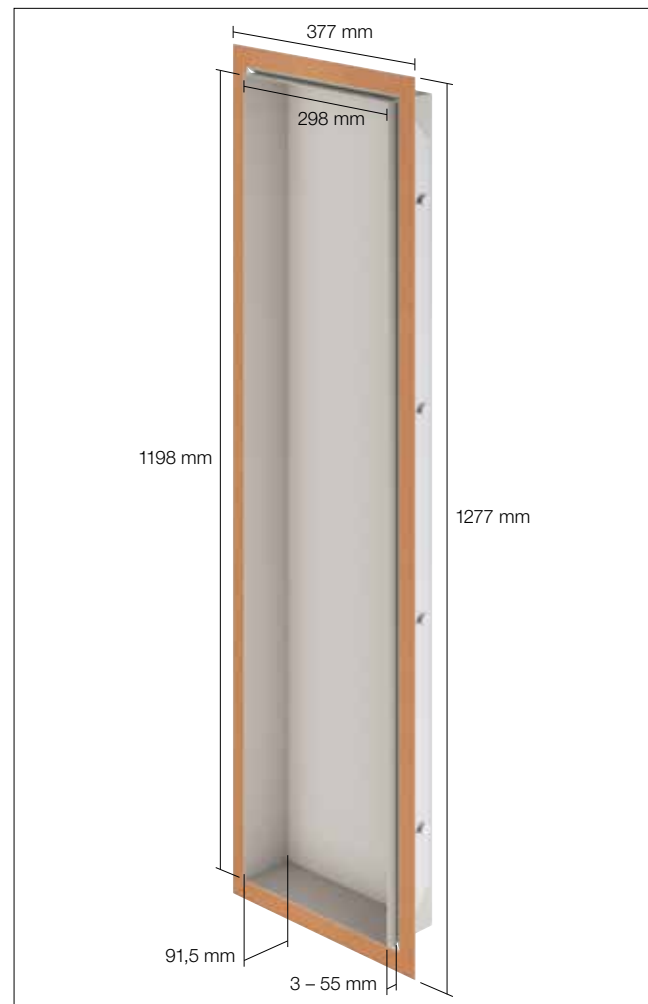
298 x 1198 mm
