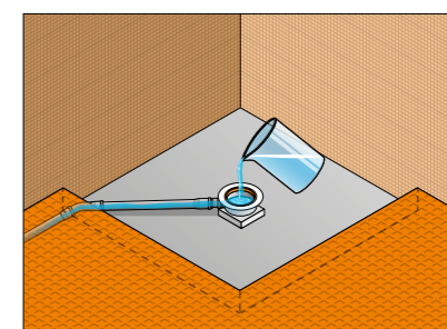
8 Dichtheitsprüfung vornehmen.
