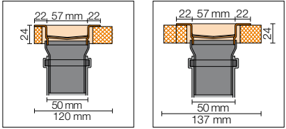
Dwarsdoorsnede wandinbouw
