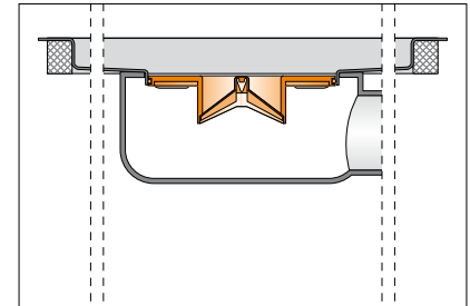
Lengtedoorsnede
