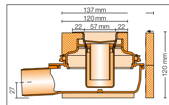
Dwarsdoorsnede
