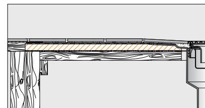
Inbouwvoorbeeld Schlüter®-KERDI-SHOWER-TT
