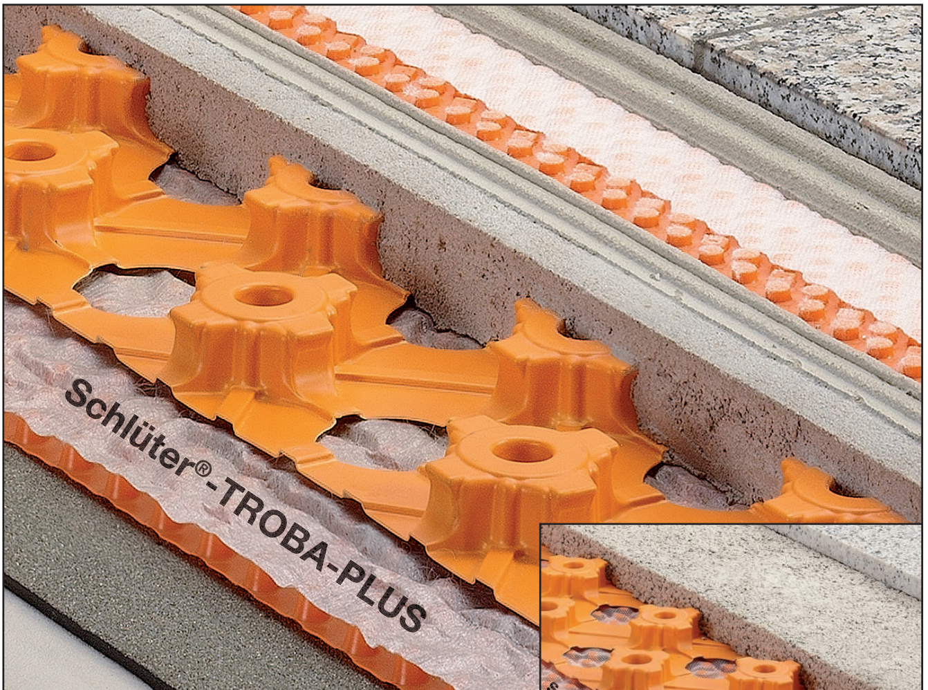
Konstruktionsaufbau mit zusätzlich obenliegender Drainagematte Schlüter®-DITRA-DRAIN.
