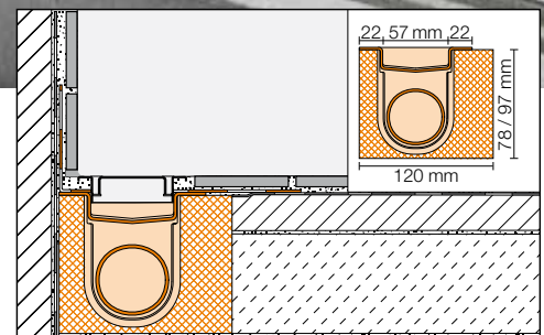
Schlüter-KERDI-LINE-H (fig. : avec cadre standard)
