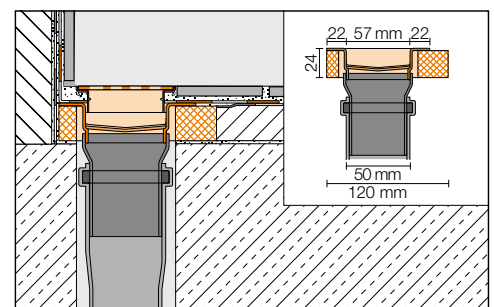
Schlüter-KERDI-LINE-V (ci-dessus avec cadre discret)
