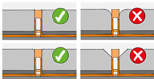
Représentation des chants de carreaux
