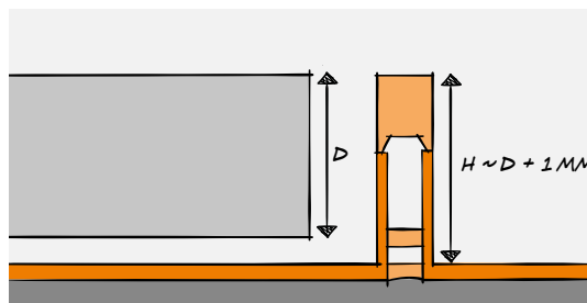
Sélectionner la hauteur du profilé en fonction de l'épaisseur du carrelage (de sorte qu'il arrive à fleur)
