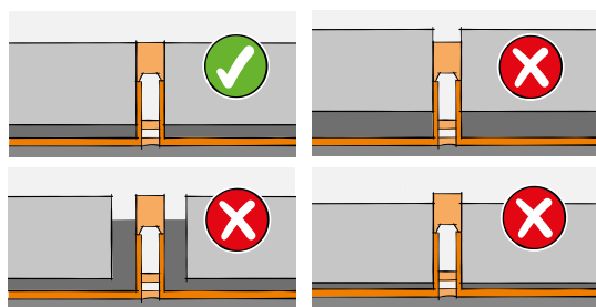
Mise en œuvre sans joint entre le profilé et le revêtement, à fleur de ce dernier.
