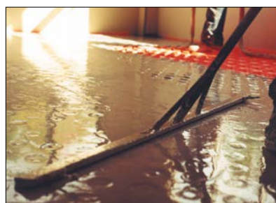
8 Alternativ zu 6 und 7 : Einbringen eines Fließestrichs auf Estrichplatte mit Folienüberzug. Um eine planebene Oberfläche zu erzielen, eignet sich z. B. das Schwabbeln mit einem groben Besen oder einer Schwabbelstange (Estrichgüte CA-C25-F4, max. F5).
