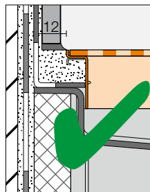
Einbau richtig (Abb. Konturrahmen)
