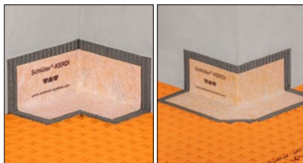
Schlüter®-KERDI-KERECK Vorgefertigte Außen- und Innenecken
