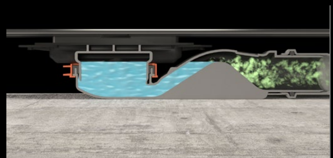
Permanenter Geruchsverschluss durch Wellenform
