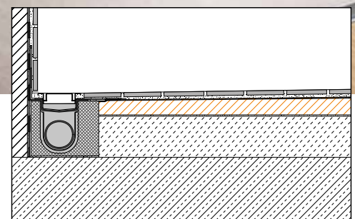
Schlüter®-KERDI-SHOWER-LTS mit Schlüter®-KERDI-LINE-H, Wandeinbau
