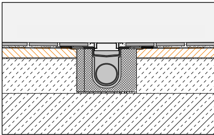
Schlüter®-KERDI-SHOWER-LT mit Schlüter®-KERDI-LINE-H, Mitteleinbau
