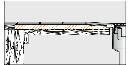
Einbaubeispiel Schlüter®-KERDI-SHOWER-TT
